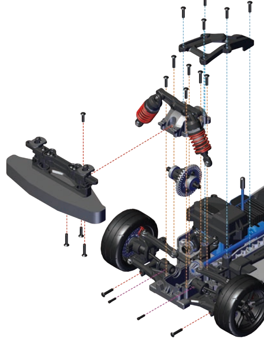
Ausbau des vorderen Differentials
